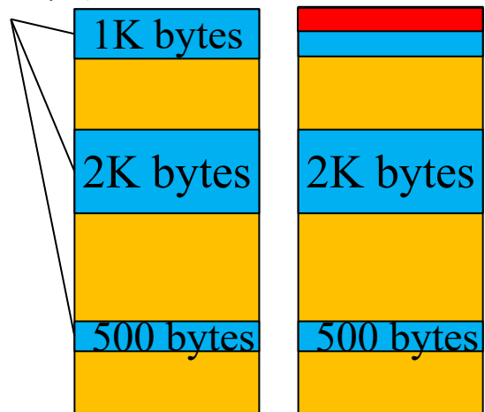
空闲块 首次分配
