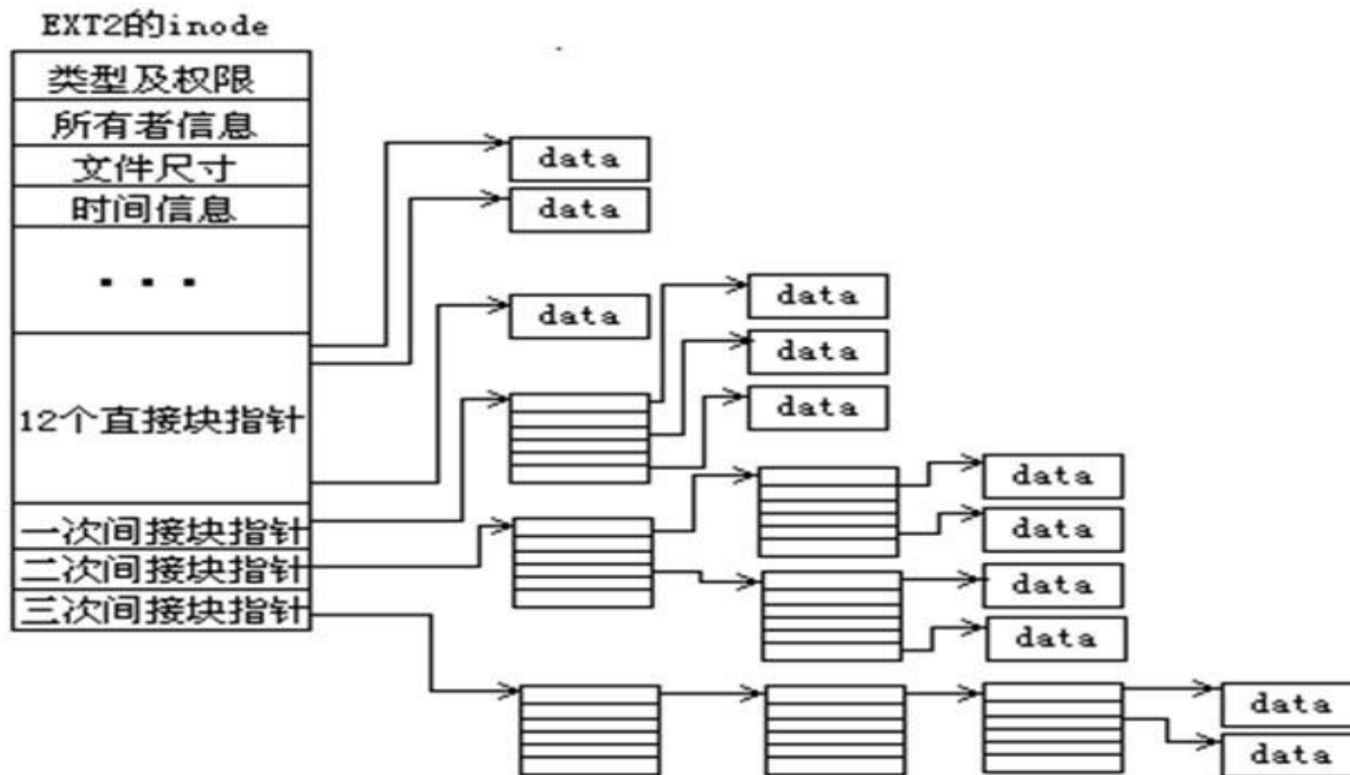
EXT2的inode中物理块指针示意图
